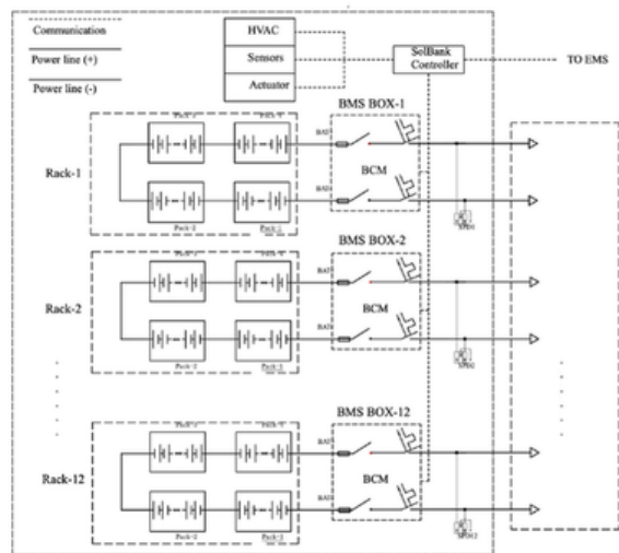
SolBank 3.0 系统电路示意图
