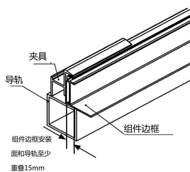
铝边框组件压块装配示意图
