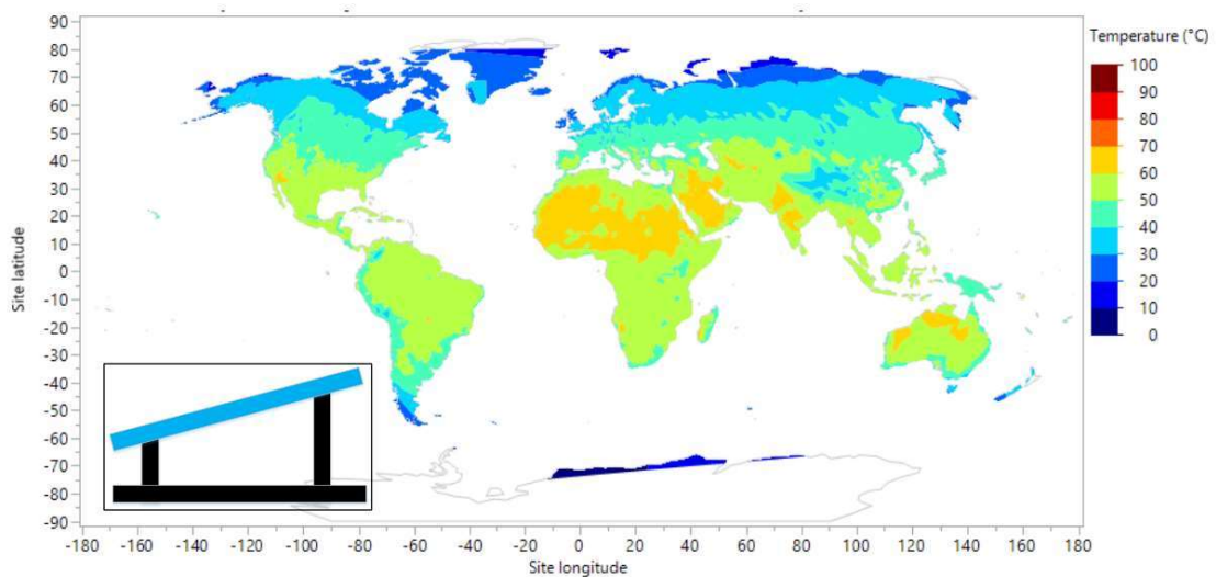
图 A.1 – 开放式支架的第 98 百分位温度分布图
