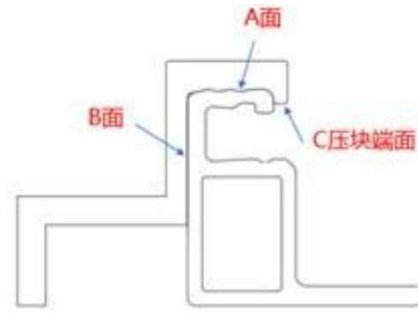
复合边框压块安装示意图
