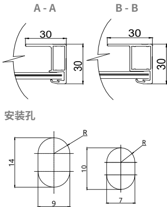
边框横截面
