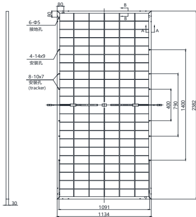
背面图
