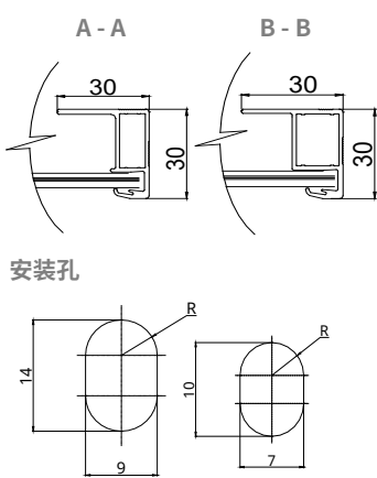
边框横截面
