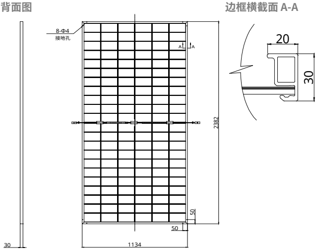
电性能参数 | STC*
