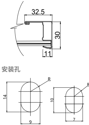
边框横截面 A - A
