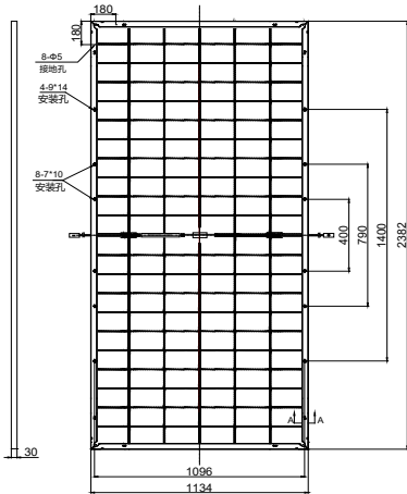
背面图
