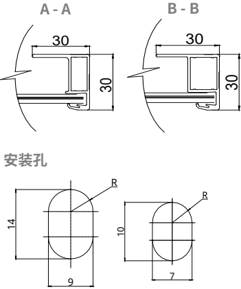
边框横截面
