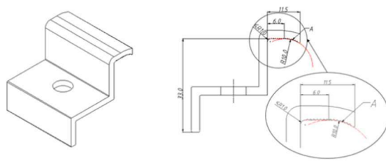
钩状压块示意图
